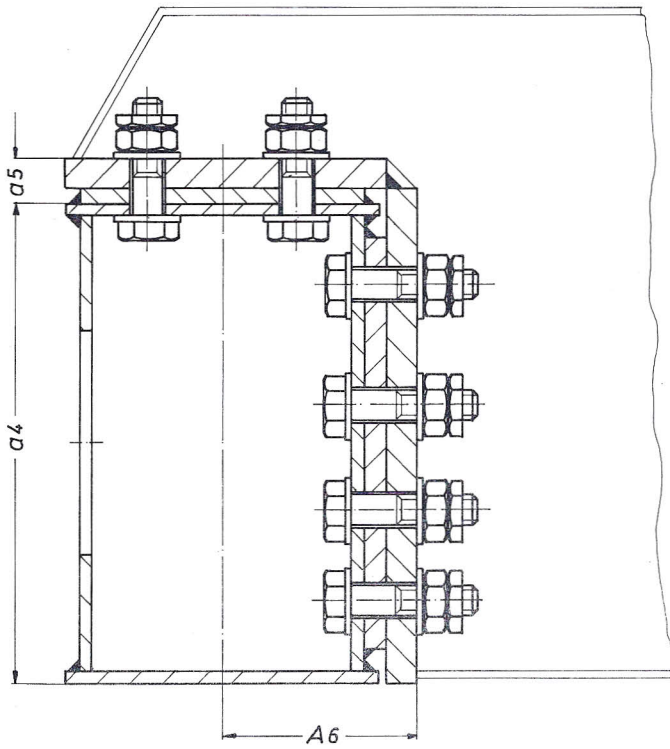
Hauptträger-Anschluß III
