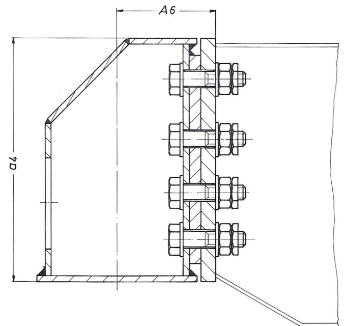
Hauptträger-Anschluß VI
