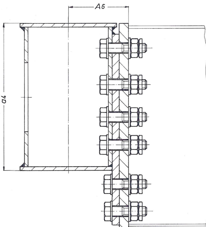
Hauptträger-Anschluß V
