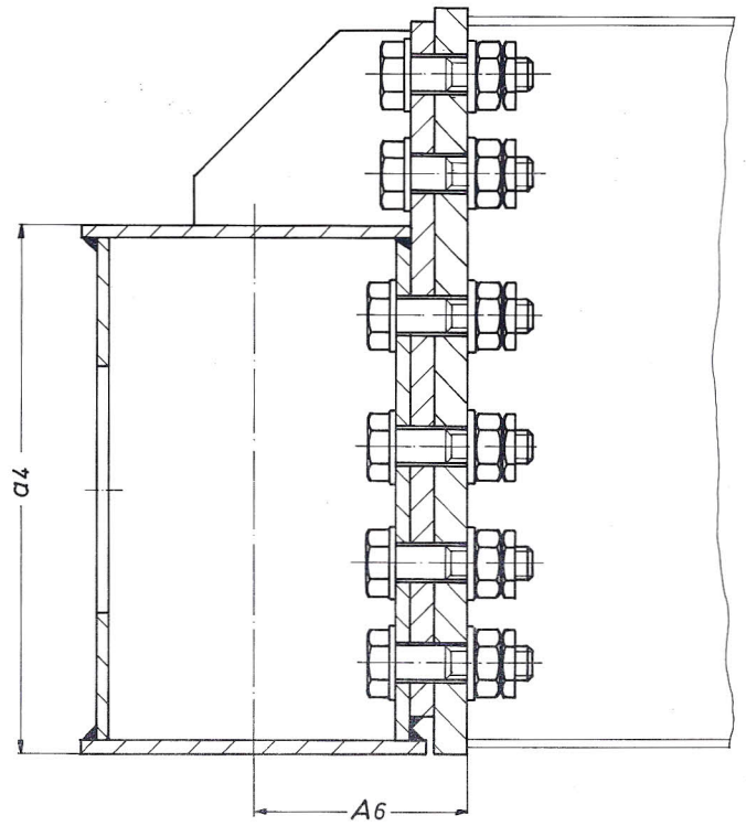
Hauptträger-Anschluß IV
